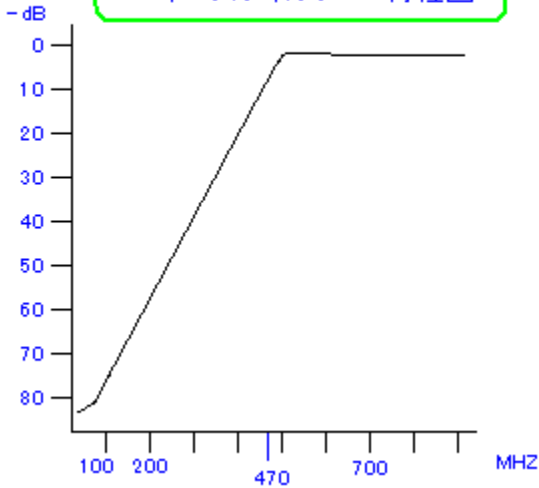
DTF-470F-HP ハイパスフィルター 特性図
