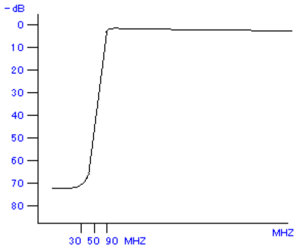
DTF-90F-HP ハイパスフィルター 特性図
